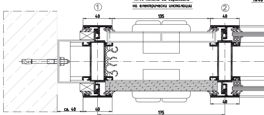
IW40 остъклено
