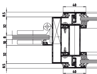
IW40 колона за вграждане на електрически инсталации
