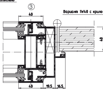
IW40 остъклено
