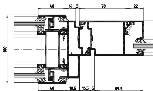
IW40 колона за вграждане на електрически инсталации
