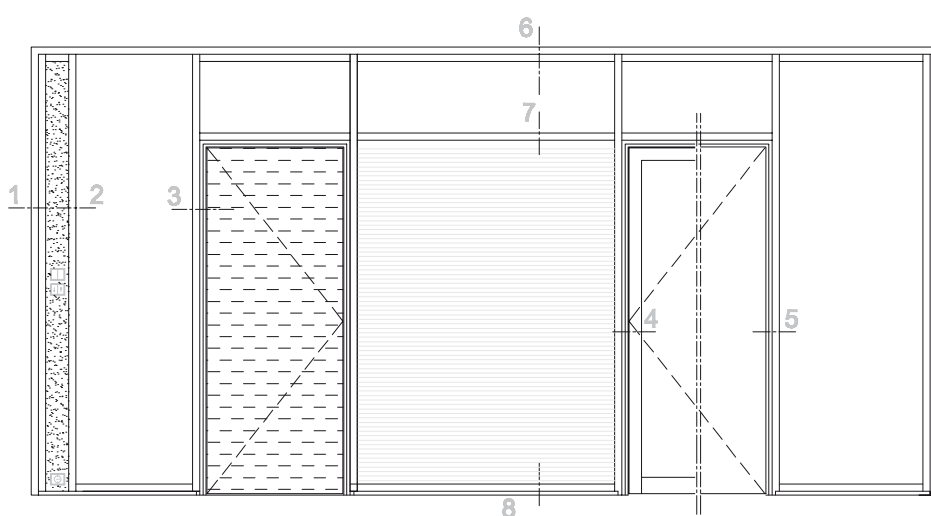
IW40 с вградена слънцезащита
